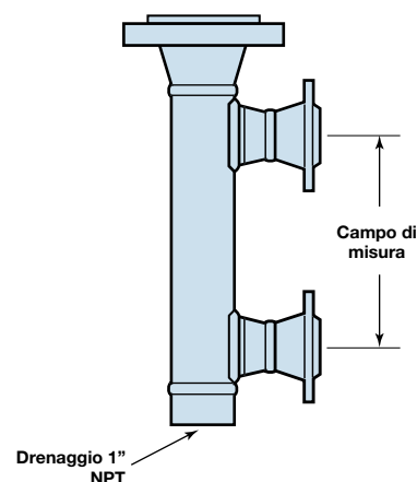
Flangia di testa con colletto saldato
